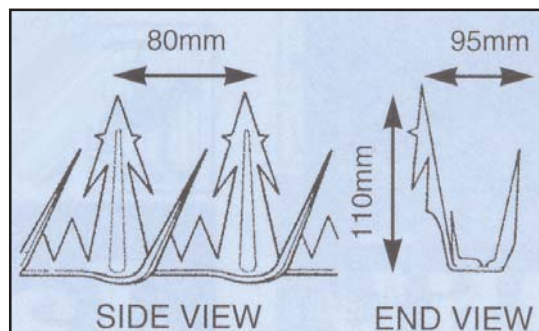
...product dimension details
